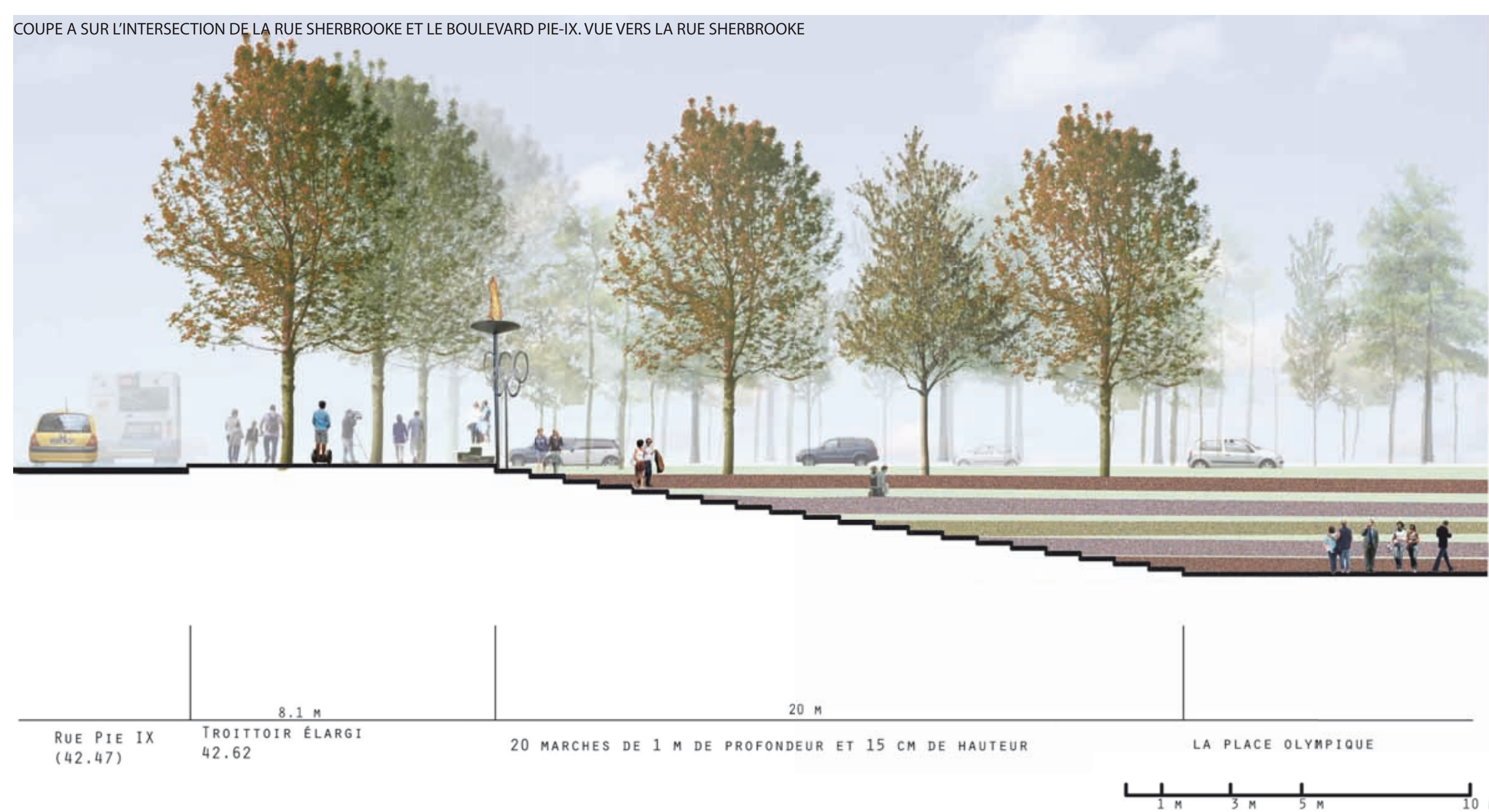
COUPE A SUR L'INTERSECTION DE LA RUE SHERBROOKE ET LE BOULEVARD PIE-IX. VUE VERS LA RUE SHERBROOKE
